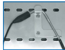
Sonda térmica con punta de silicona
