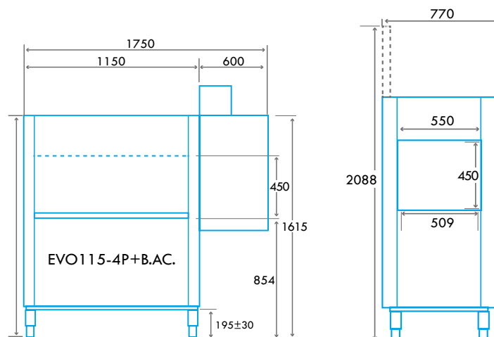
EVO115-4P+BOMBA ACLARADO MESAS DE ENTRADA Y SALIDA OPCIONALES
