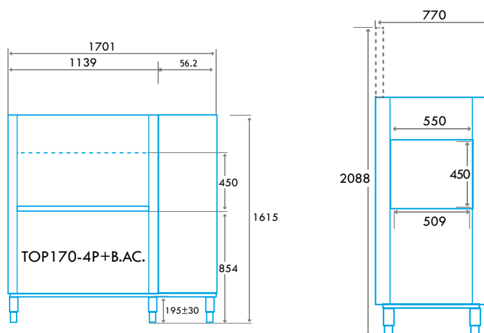
TOP170-4P + BOMBA ACLARADO MESAS DE ENTRADA Y SALIDA OPCIONALES
