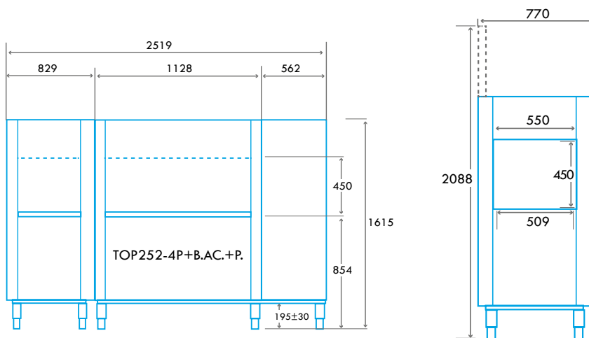
TOP252-4P+B. ACLARADO+PRELAVADO MESAS DE ENTRADA Y SALIDA OPCIONALES
