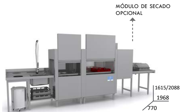
EVO197-4P+B. ACLARADO+PRELAVADO
